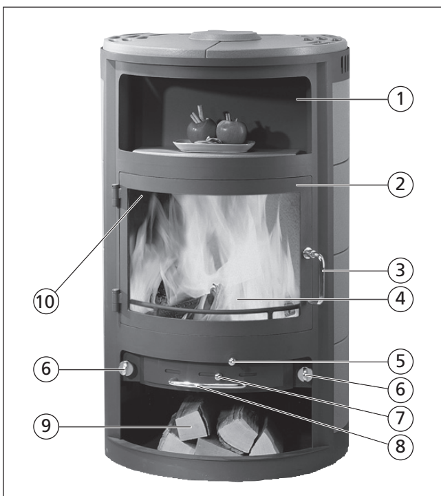
Raumheizer/Kaminofen »Hamburg II«
