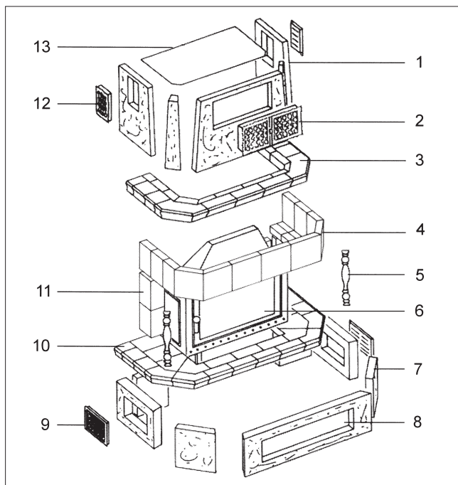
2-1 Kaminelemente, Variante Kachelverkleidung
