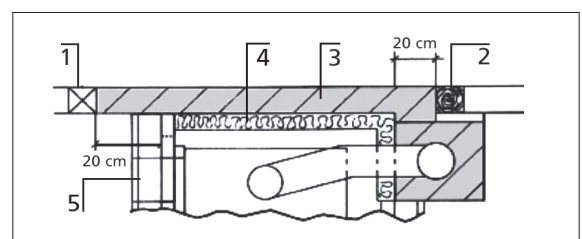
Bild 1-1 vollflächige Brandschutzwand
