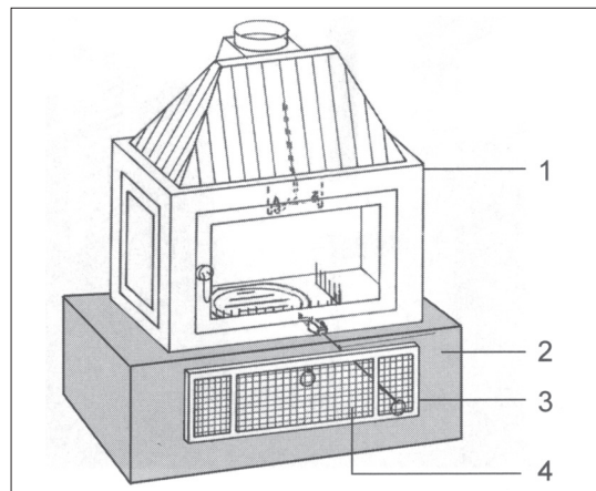
Bild 2-8 Sockel mit Zuluftöffnung
