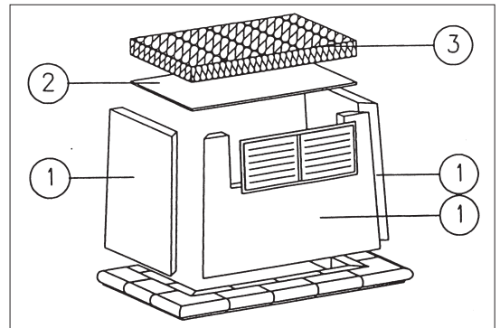
1 Gießschamotte-Module 2 Dämmplatte mit Alukaschierung 3 Mineralwolle
