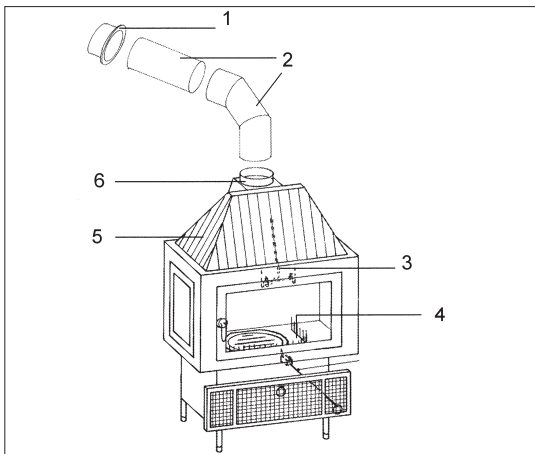
Bild 2-10 Kamineinsatz/Verrohrung
