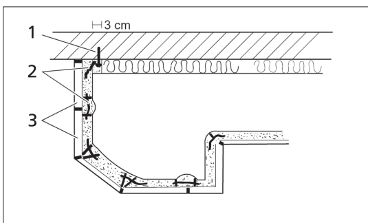
Bild 2-11 Wandanschluss, Drähte befestigen
