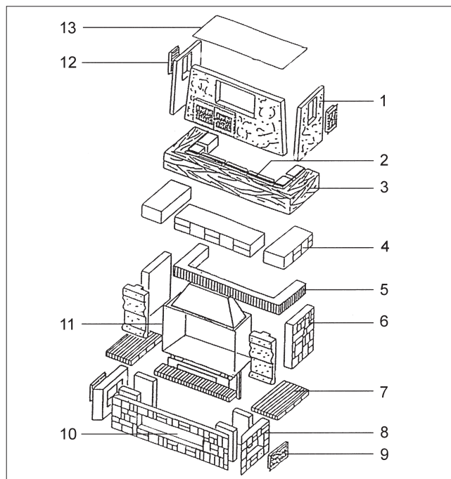
2-2 Kaminelemente, Variante Naturstein
