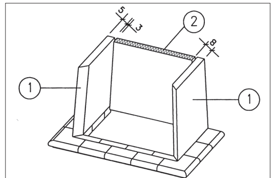
1 Gießschamotte 2 Dämmplatte
