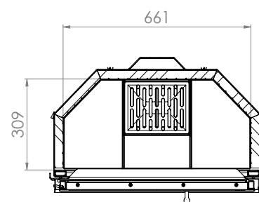
PRZĘKRÓJ A-A
